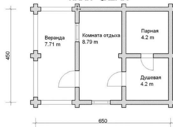
ПЛАН - СХЕМА
