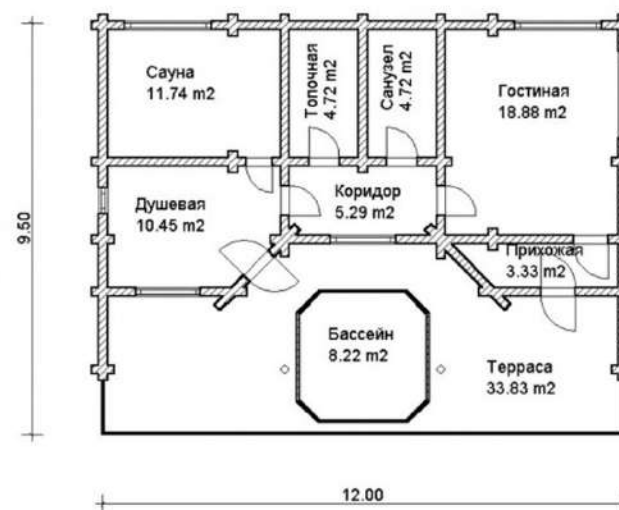
ПЛАН - СХЕМА
