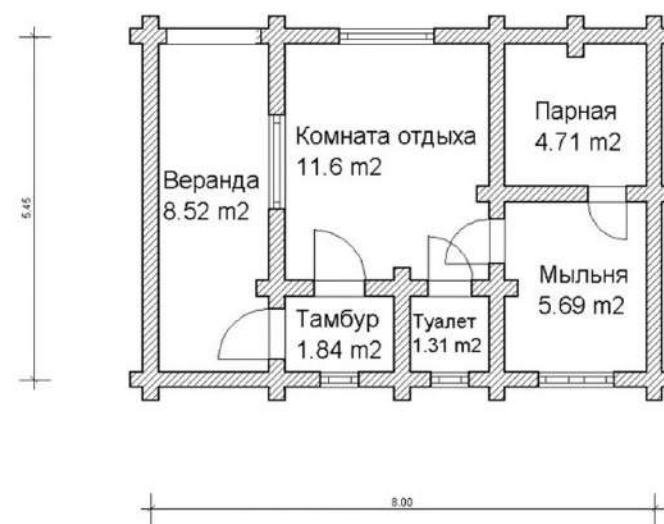
ПЛАН - СХЕМА
