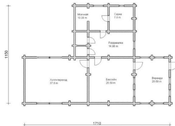
ПЛАН - СХЕМА
