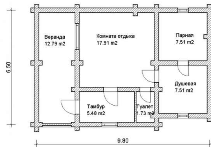
ПЛАН - СХЕМА
