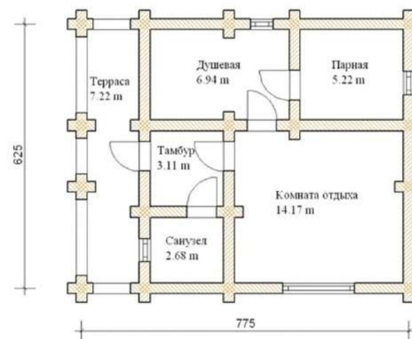
ПЛАН - СХЕМА
