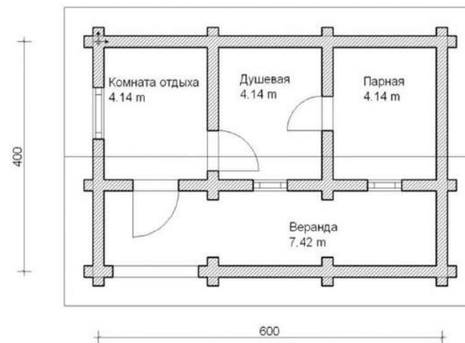
ПЛАН - СХЕМА
