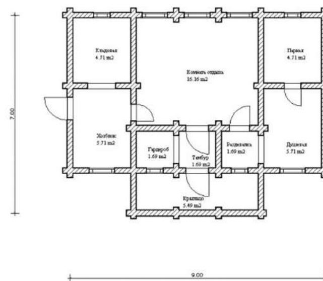
ПЛАН - СХЕМА
