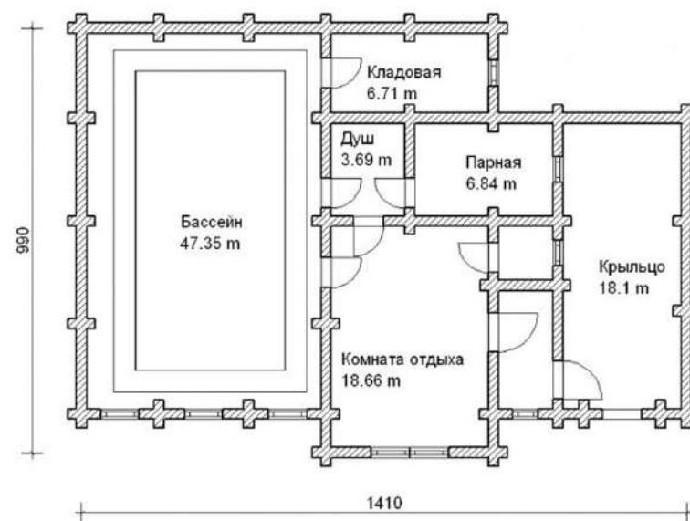
ПЛАН - СХЕМА
