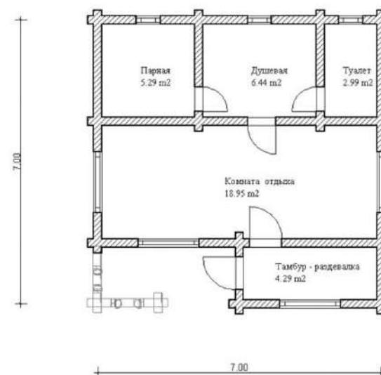
ПЛАН - СХЕМА
