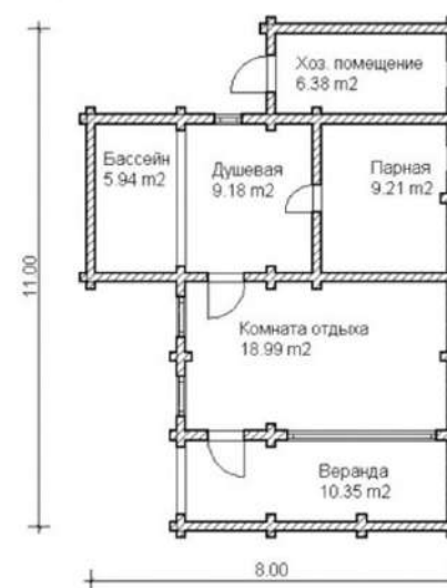
ПЛАН - СХЕМА
