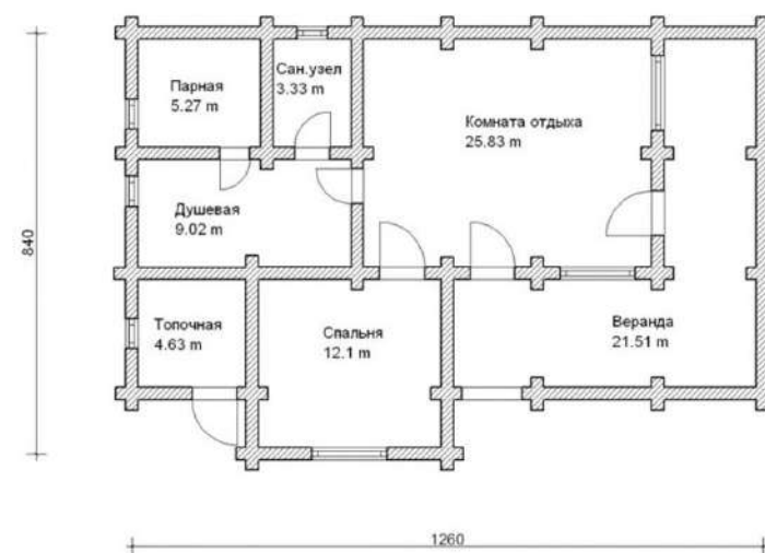
ПЛАН - СХЕМА
