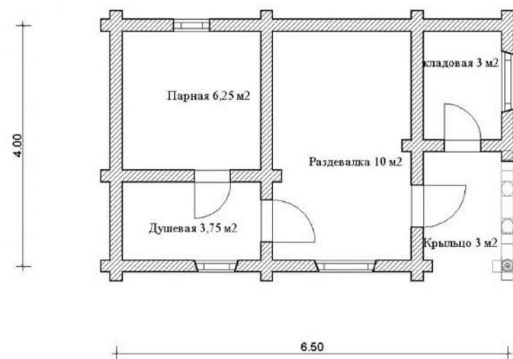
ПЛАН - СХЕМА
