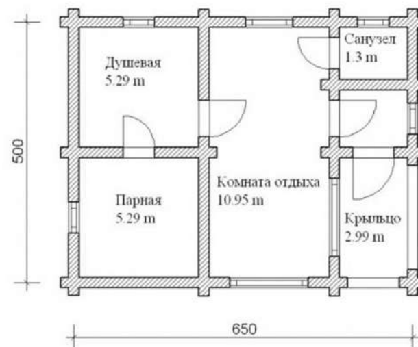
ПЛАН - СХЕМА
