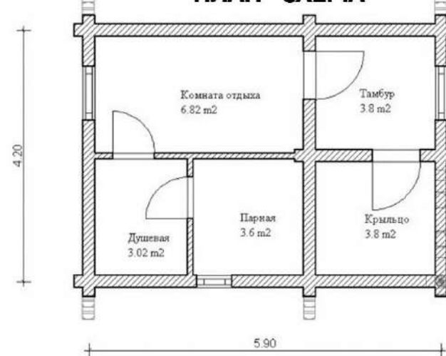
ПЛАН - СХЕМА
