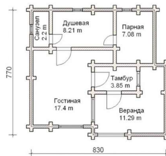
ПЛАН - СХЕМА
