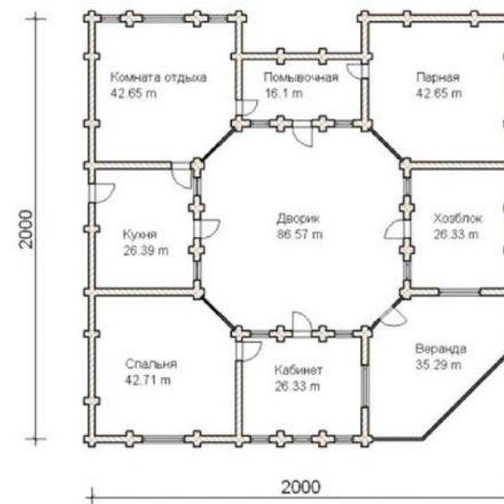
ПЛАН - СХЕМА
